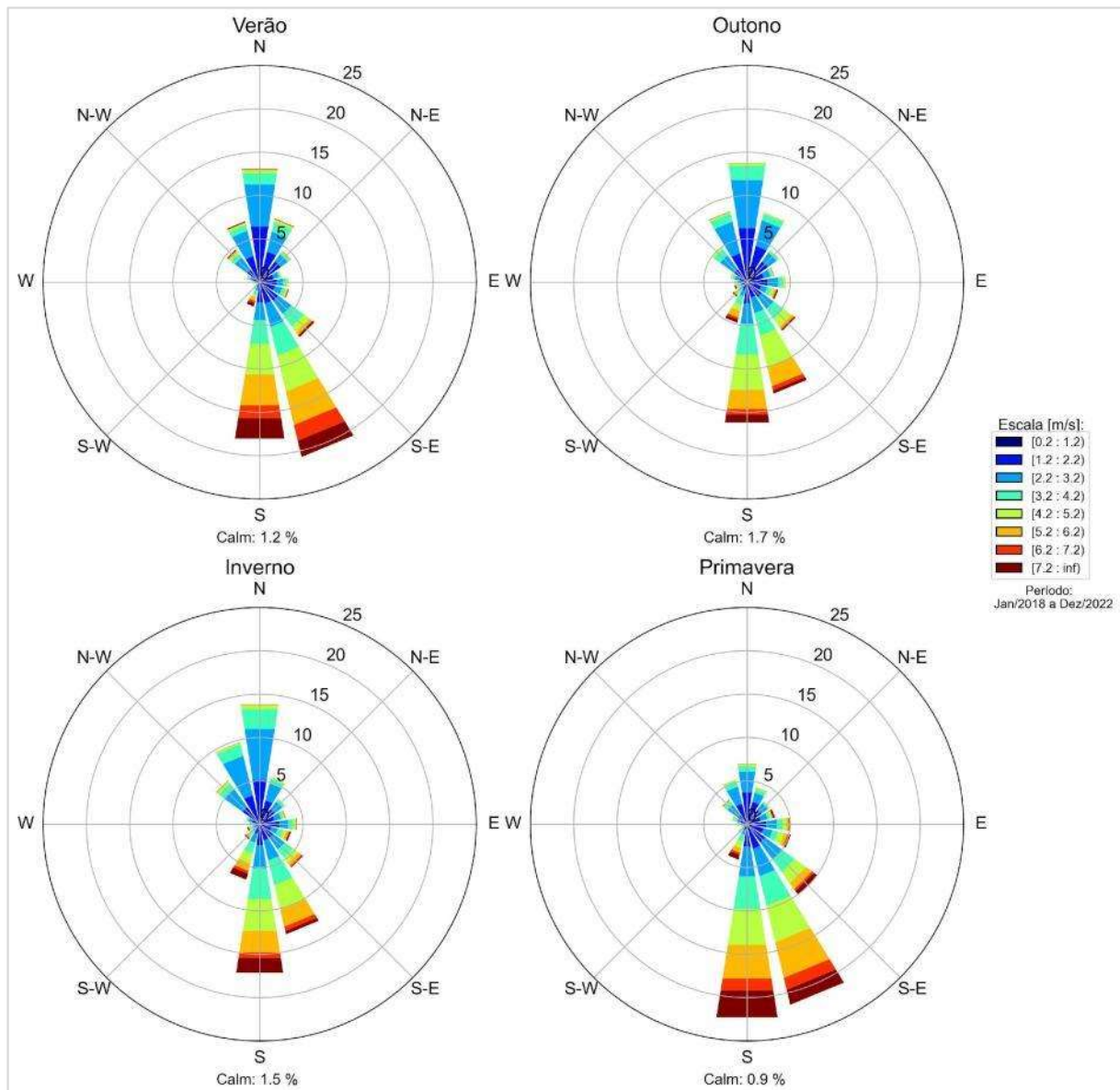
Figura 3.2 Rosas dos ventos sazonais do Aeroporto Santos Dumont no período de janeiro de 2018 a dezembro de 2022.
