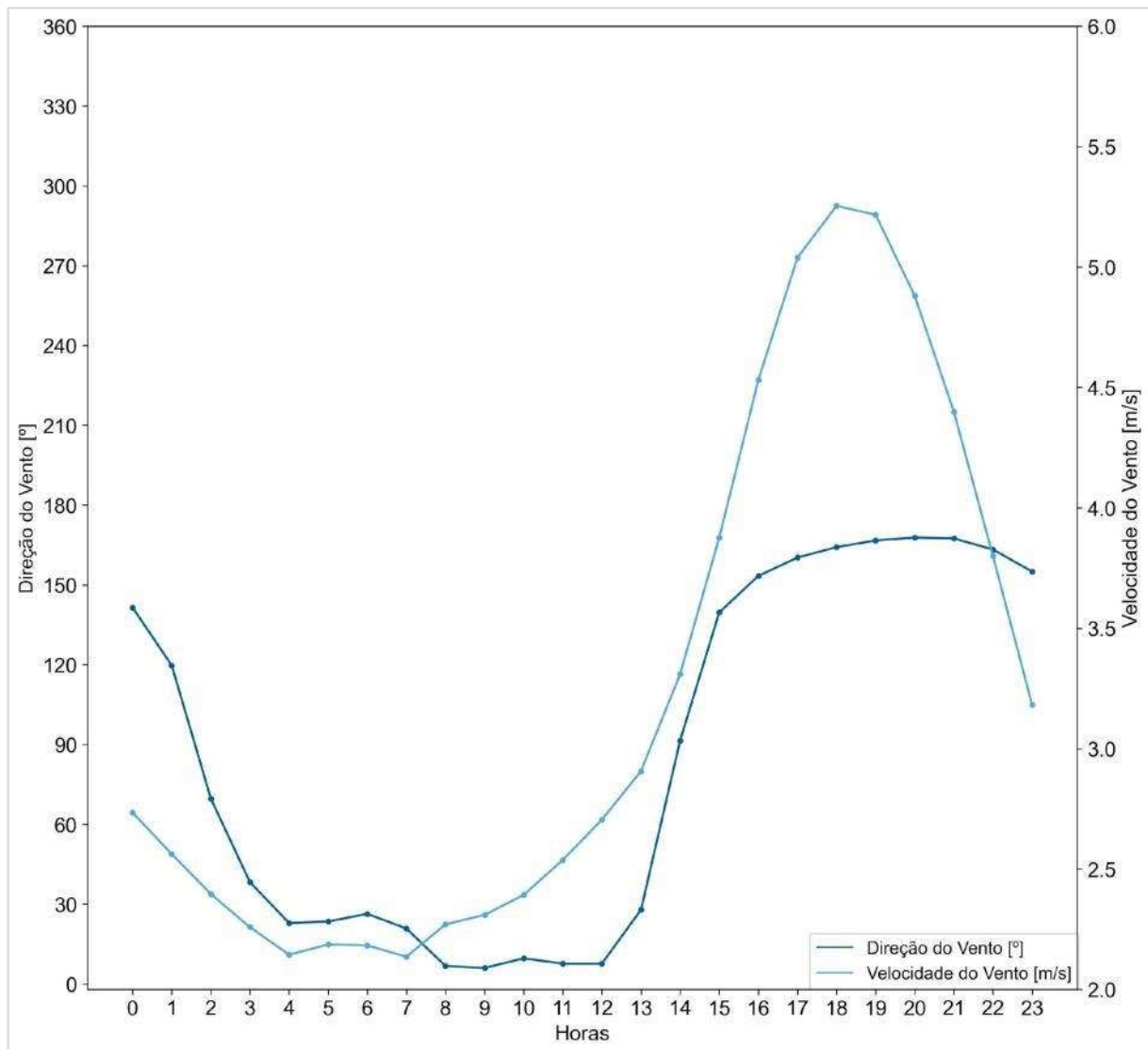
Figura 3.3 Gráfico da média horária da direção e velocidade do vento dos dados do Aeroporto Santos Dumont no período de janeiro de 2018 a dezembro de 2022.
