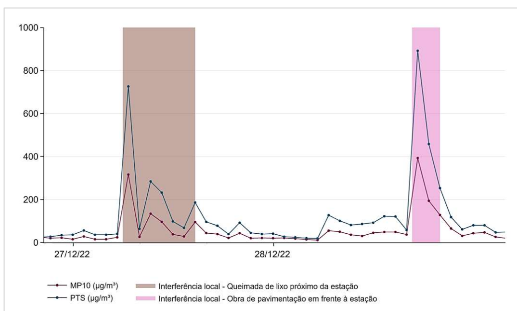
Figura 3.6 Gráfico de linhas de monitoramento de PTS e MP 10 .
