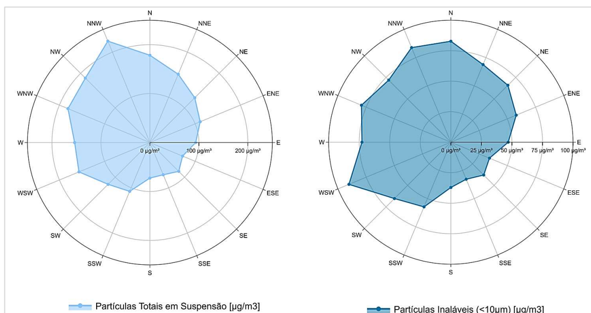
Figura 3.8 Radares de poluente de PTS e MP 10 .
