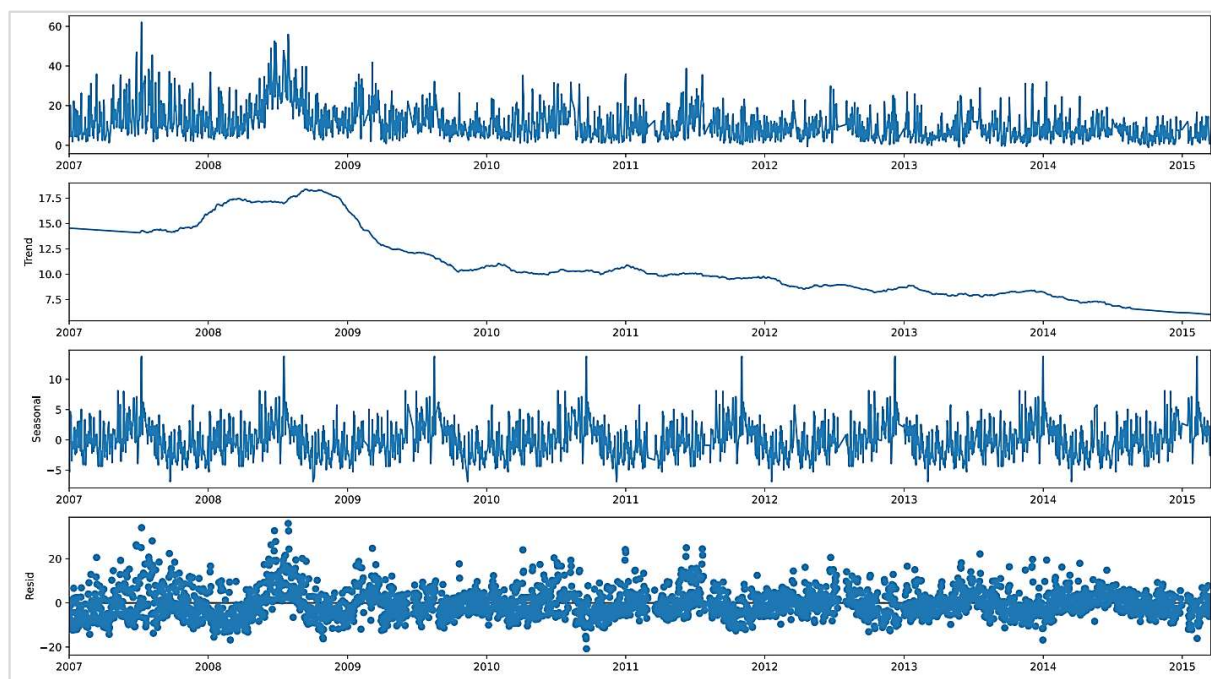
Figura 3.9 Decomposição de dados do monitoramento de MP_{2,5} da cidade de Nova Jersey (Nova Iorque, EUA) - Estação 34-017-1003 (2007 a 2015).
