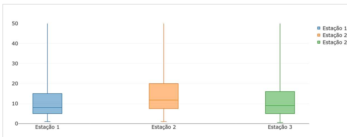
Figura 3.7 Box plot referente ao monitoramento de MP_{2,5} em três estações numa mesma localidade.
