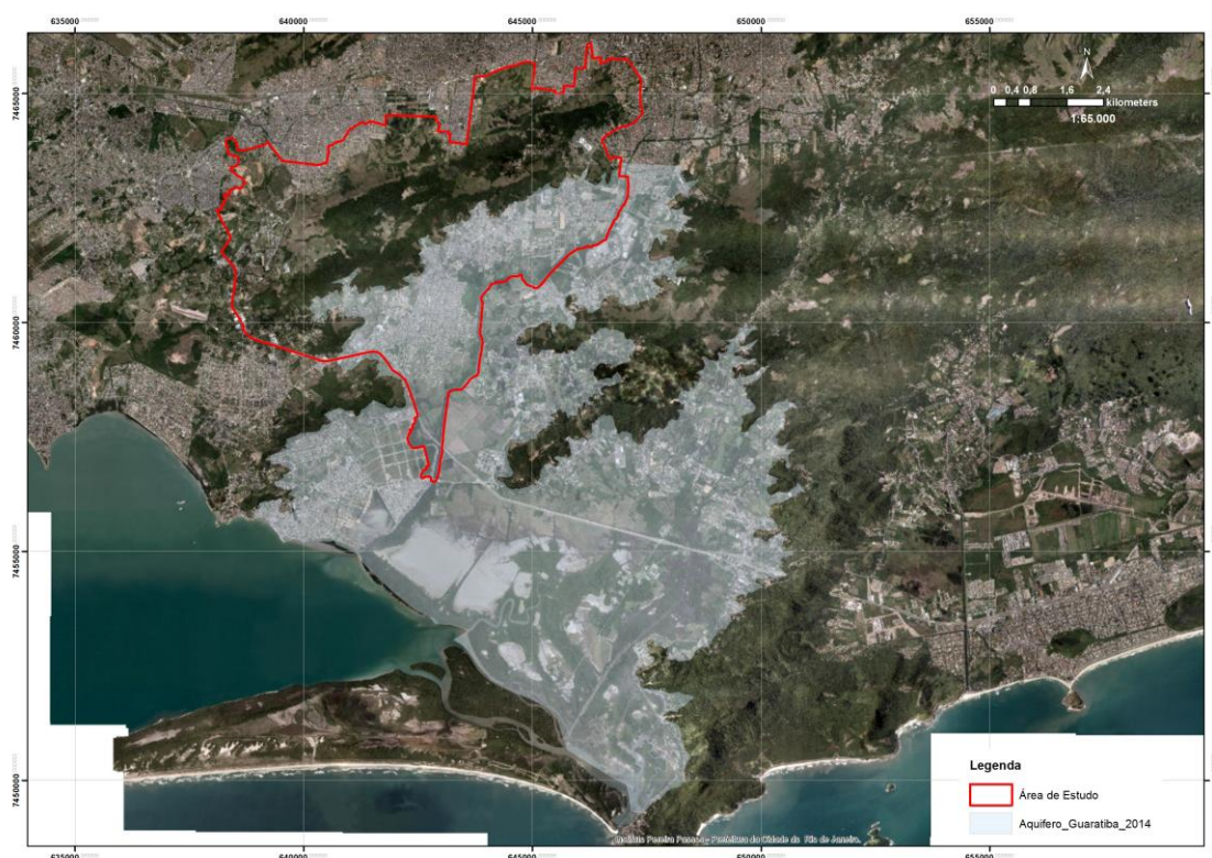
Figura 8 – Limite do aquífero Guaratiba, delimitado no âmbito do grupo de pesquisa coordenado pela professora dra Maria Geralda do departamento de geociências da UFRJ. Elaborado por PCRJ/SMA/CGMA/GMFA7.
