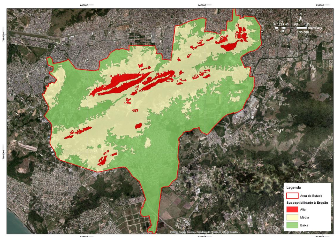
Figura 19 – Mapa de susceptibilidade à erosão dos solos da área de estudo. Fonte: Fundação GeoRio (1997). Elaborado por PCRJ/SMA/CGMA/GMFA7.
