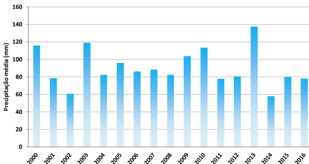
Figura 5 - Precipitação média mensal (em milímetros) para um período de 16 anos (2000 – 2016). PCRJ – SCMA/CGMA/GEPA - Fonte: GEO-Rio e INMET.
