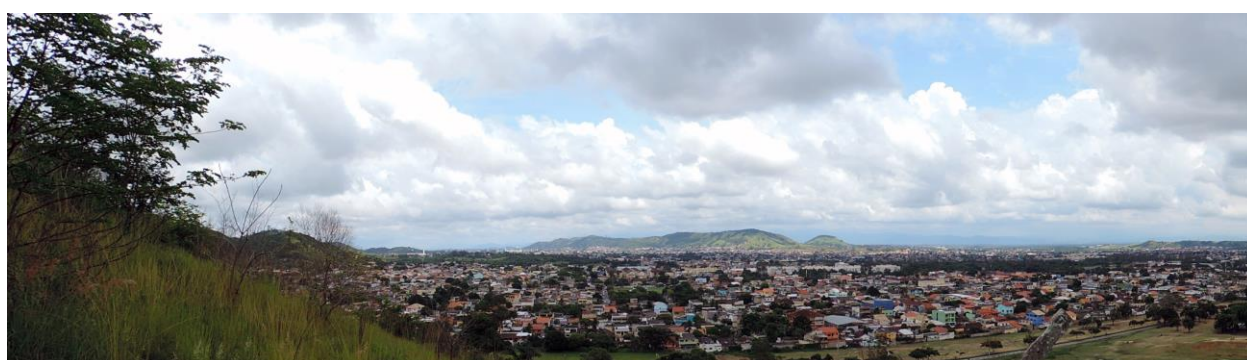
Figura 81 – Panorama visualizado a partir do Reservatório. Foto: Vladimir da Franca Fernandes.
