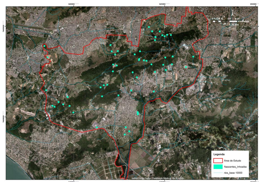
Figura 23 – Mapa de nascentes existentes na área de estudo. Elaborado por PCRJ/SMA/CGMA/GMFA7.
