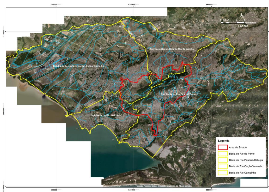
Figura 21 – Mapa das bacias hidrográficas abrangidas pela área de estudo. Elaborado por PCRJ/SMA/CGMA/GMFA7
