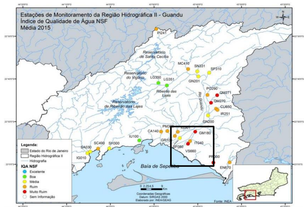
Figura 25 – Mapa com a localização dos pontos de monitoramento da qualidade da água realizados pelo INEA, destacados no quadrado os pontos PR000 do Rio Piraquê-Cabuçu e IT040 do Canal do Itá. Constata-se IQA classificado como ruim para o ponto IT040 e muito ruim para o ponto PR000, no ano de 2015. Elaborado por PCRJ/SMA/CGMA/GMFA6.
