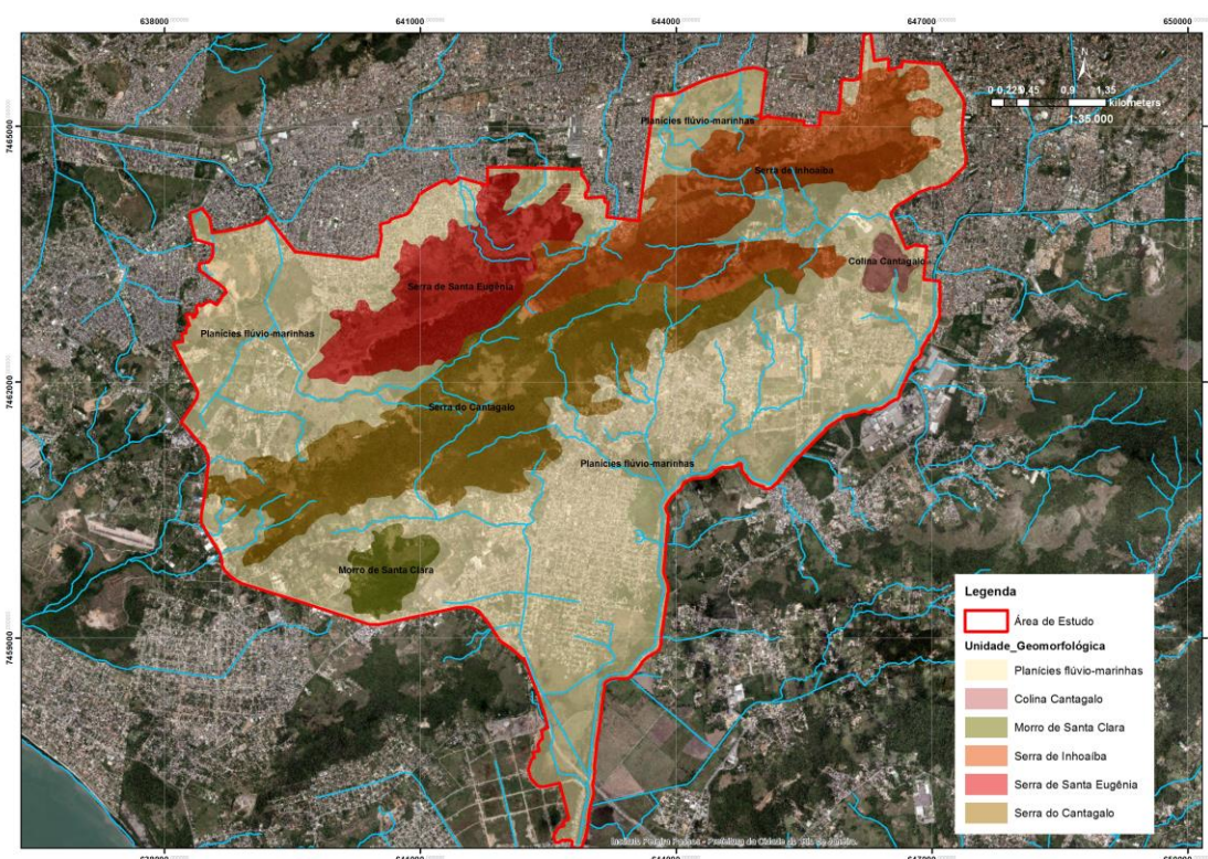
Figura 9 – Mapa Geomorfológico da área de estudo. Adaptado da base geomorfológica do Estado do Rio, disponibilizado pelo INEA. Elaborado por PCRJ/SMA/CGMA/GMFA7.
