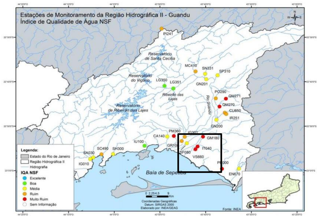
Figura 24 – Mapa com a localização dos pontos de monitoramento da qualidade da água realizados pelo INEA, destacados no quadrado os pontos PR000 do Rio Piraquê-Cabuçu e IT040 do Canal do Itá, ambos apresentando Índices de Qualidade da Água (IQA) muito ruins para o ano de 2014. Elaborado por PCRJ/SMA/CGMA/GMFA6.
