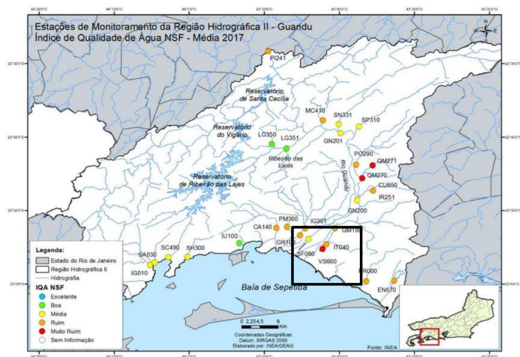
Figura 27 – Mapa com a localização dos pontos de monitoramento da qualidade da água realizados pelo INEA, destacados no quadrado os pontos PR000 do Rio Piraquê-Cabuçu e IT040 do Canal do Itá, ambos apresentando Índices de Qualidade da Água (IQA) ruins para o ano de 2017. Elaborado por PCRJ/SMA/CGMA/GMFA6.
